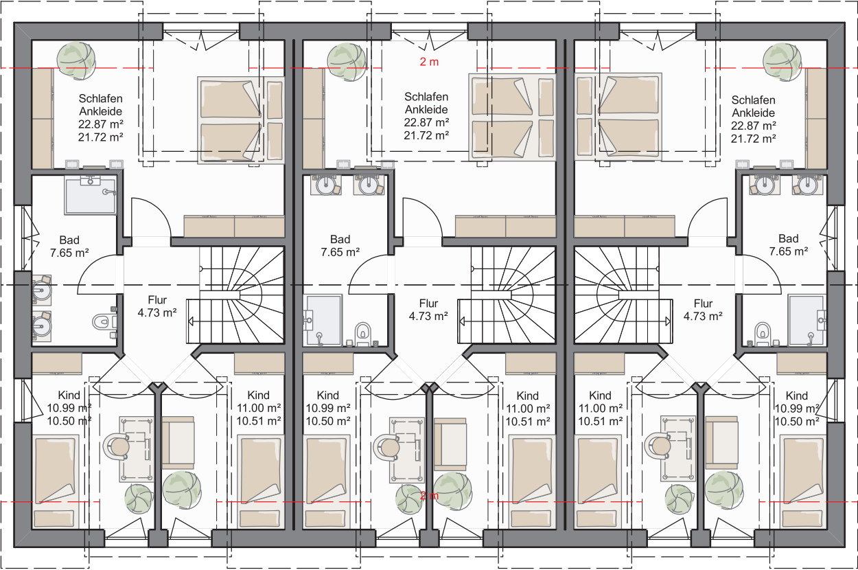
Grundriss DG
